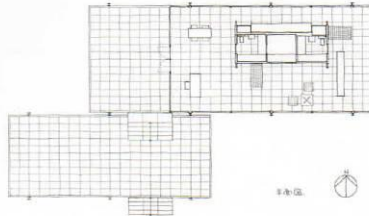
ファンズワース邸—アメリカ
