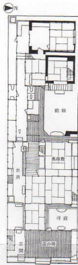
京都の町家—吉田家 1階 平面図
