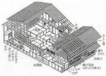
京都の町家—表屋造り
